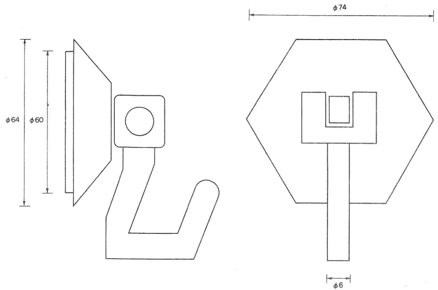
φ60フンタッチフックGPPSET HOOK-60-GPP
