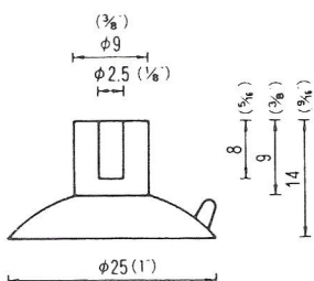
φ25立穴φ2.5 QT-25-2.5 5,000PCS
