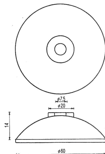
φ70引張り用アダプター AD-70-PL-W USE QPUL-70 500ヶ
