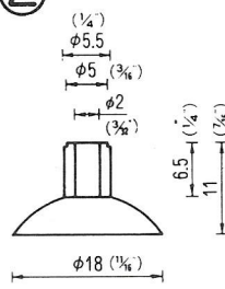
φ18立穴φ2 QT-18-2 5,000PCS
