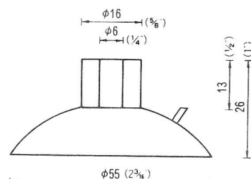
φ55立穴φ6(引張ベロ付) QT-55-6 1,000PCS
