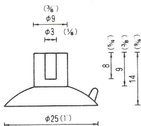
φ25立穴φ3 QT-25-3 QT-25-4
