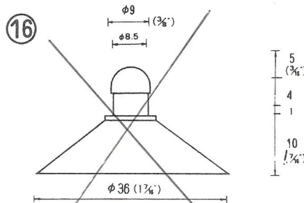
φ36横溝ドームヘッド QM-36-DH 2,500PCS
