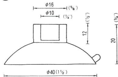
φ40立穴φ10 QT-40-10 2,000PCS
