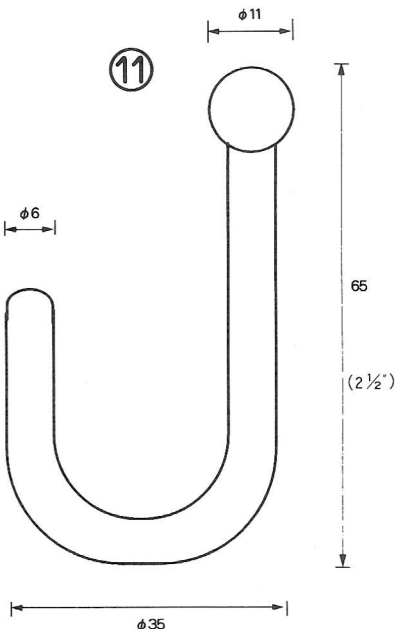
55Jフック HOOK-55-J
