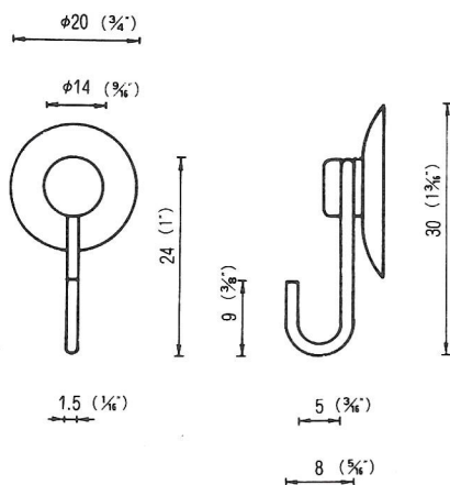
φ20線材フック HOOK-20-IR (受注生産品) 特注ロット 10,000ヶ以上 COSTOM MADE OVER 10,000pcs
