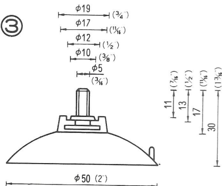
φ50 インサート吸着盤-GPP ネジ径 5m/m六角ナット使用 QSC-50-5-GPP(受注生産品) 1,000PCS
