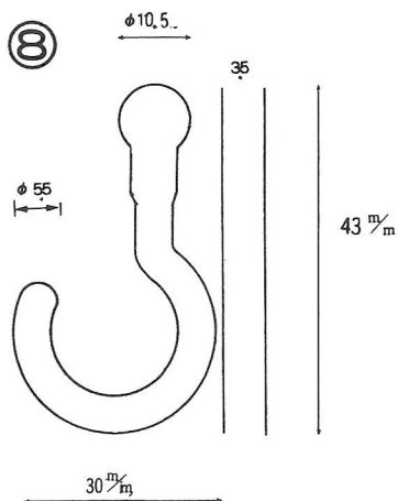
サンゴーフック薄型トーマー HOOK-35-UT For QY-35 (受注生産品)
