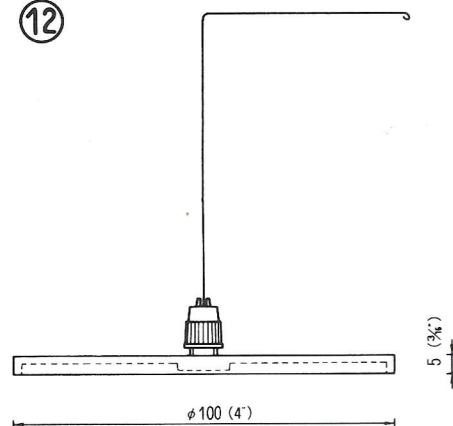
φ100 円盤 (ABS) プラチャック付 AD-100-WP 線材立て用
