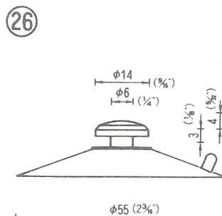
φ55横溝キッチン QM-55-K ※ 2,000PCS
