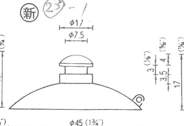
φ45横溝φ17 QM-45-17 2,000PCS (塩ビ：受注生産品 脱塩ビ：成形不可)
