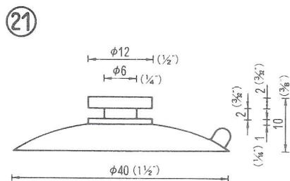
φ40横溝キッチン QM-40-K 2,500PCS
