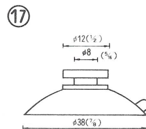
φ38横溝 QM-38 2,500PCS (脱塩ビ：受注生産品)
