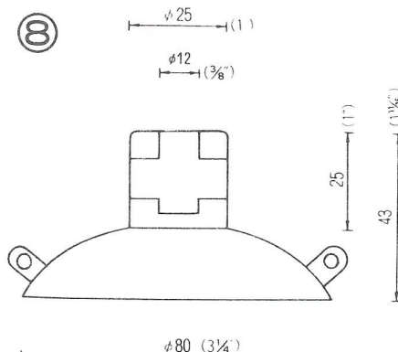
φ80立横穴φ12シボ QTY-80-12SB ※ 200PCS (脱塩ビ：受注生産品)
