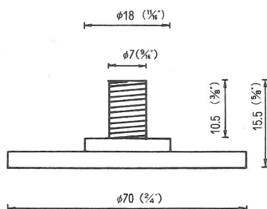
φ70引張り吸着盤 GPP QPUL-70-GPP ※500PCS
