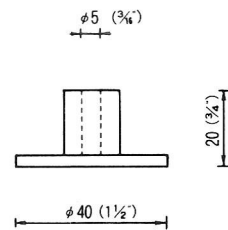
φ40/パネ立て サンゴーヒンジをパネに セットしてφ5の穴に 差し込みます。 AD-40 ABS (受注生産品)
