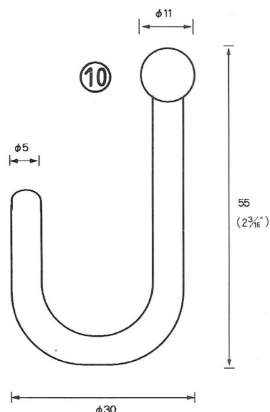
40Jフック HOOK-40-J
