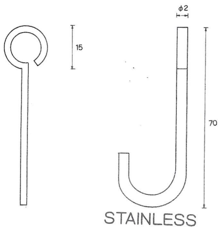
ステンレス70フックφ2 HOOK-70-ST For QPUL-45
