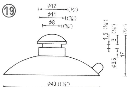
φ40横溝シボ QM-40-SB 2,500PCS (脱塩ビ：受注生産品)
