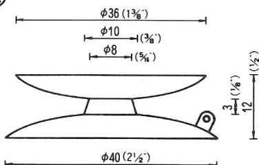
φ40 両面吸着盤 Both Type R-40 QR-40 ※ 2,000PCS
