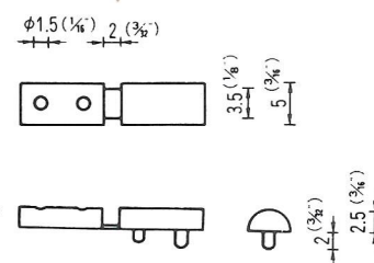
サンゴーヒンジバネ AD-ST-35S 穴径φ5に使用可
