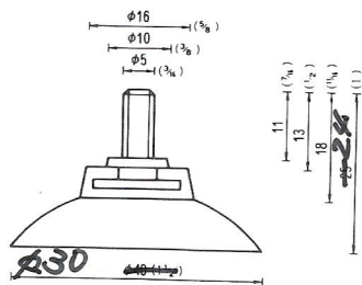
φ30インサート吸着盤GPP ネジ径5% 六角ナット使用 QSC-30-5-GPP 2,000PCS (受注生産品)
