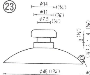
φ45横溝シボ QM-45-SB 2,000PCS (受注生産品)
