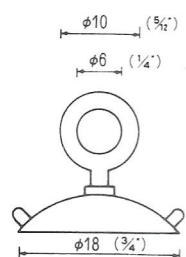
φ18横穴φ6ホース QHS-18-6 (鑑賞用水槽の ホース押えに！) 5,000PCS (脱塩ビ：受注生産品)
