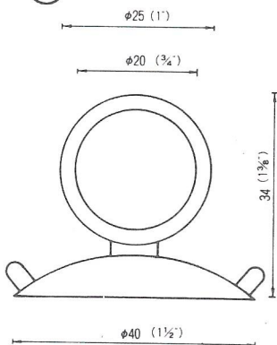
φ40横穴φ20ホース QHS-40-20 1,500PCS (脱塩ビ：受注生産品)
