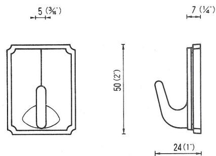
フロントフック 両面テープ付 WB-T-FL 特注ロット 10,000ヶ以上 COSTOM MADE OVER 10,000pcs
