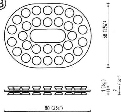
石ケン用小判吸着盤 QR-SOAP ※ 500PCS
