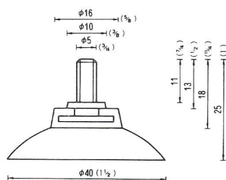
φ40インサート吸着盤GPP ネジ径5% 六角ナット使用 QSC-40-5-GPP 2,000PCS (受注生産品)
