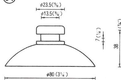
φ80横溝 QM-80 ※ 200PCS (脱塩ビ:成形不可)
