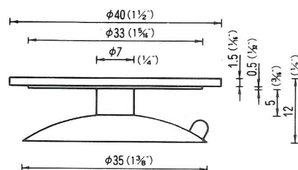
φ35 ウェルダー QW-35 ※ 2,000PCS
