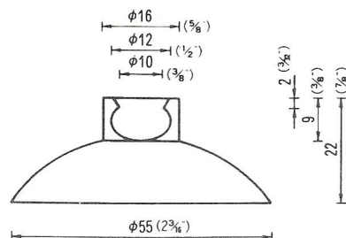
φ55立穴φ12玉入 QT-55-B12 1,000PCS (受注生産品)
