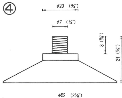
φ52インサート吸着盤シボ-GPP QSC-52-7-SB-GPP 1,500PCS
