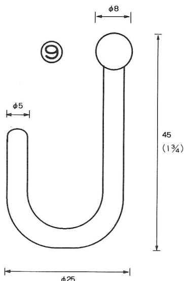
ヨンゴーフック 穴あき HOOK-45-H For QY-45
