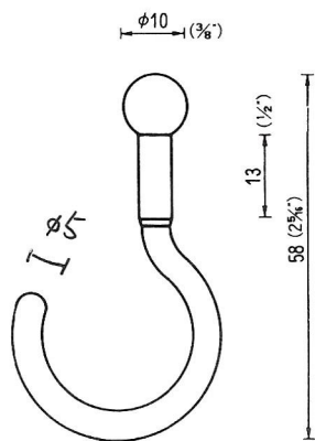
ヨンゴーフック For QY-45 1½, 1¾" SIDEHOLE HOOK-45
