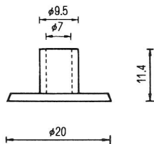
φ20/パネ立て アダプター-50が入ります。 AD-20 ABS (受注生産品)
