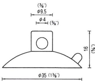
φ35横穴φ4 QY-35-4 2,500PCS
