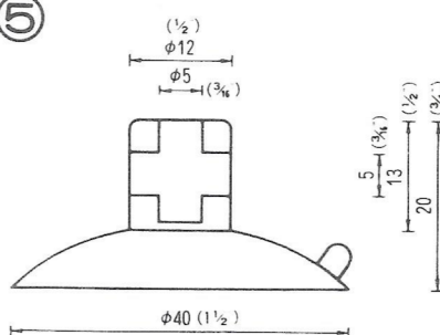
φ40立横穴φ5シボ QTY-40-5SB 2,500PCS (脱塩ビ：受注生産品)
