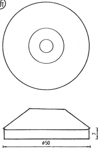
φ55引張り用アダプター AD-55-PL-W USE QPUL-55 1,000ヶ
