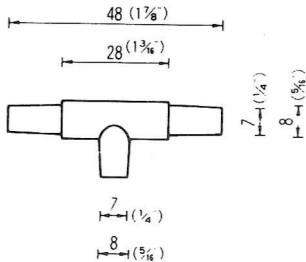
T字バネスティ(白) AD-ST-T-W 2,000ヶ
